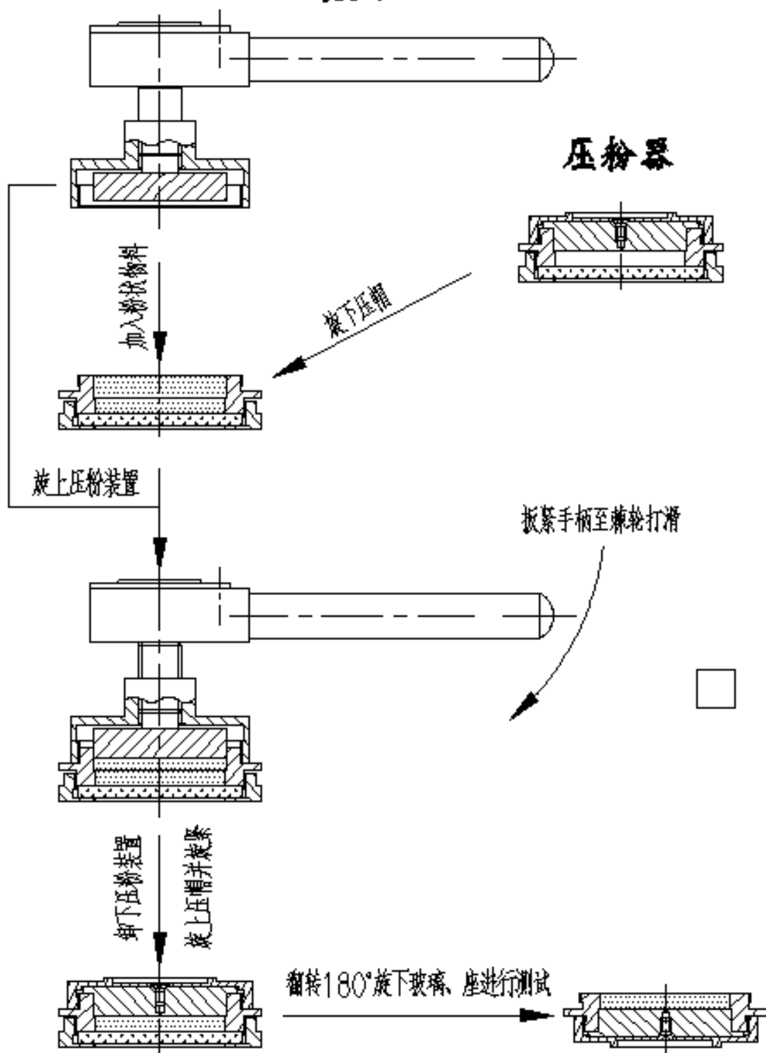
恒压取样器操作示意图
